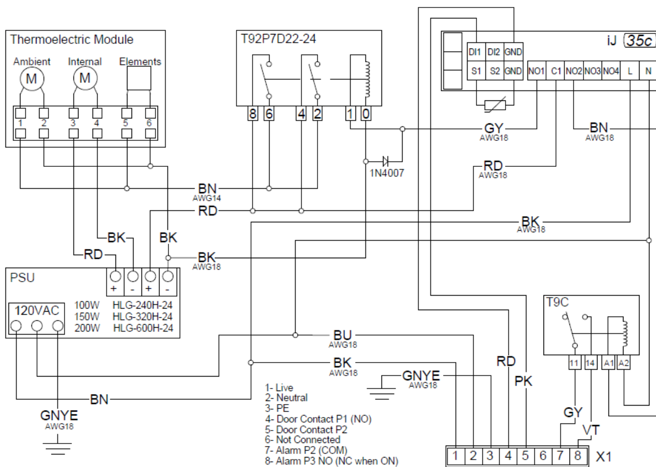
100W / 150W / 200W TE Wiring Diagram 596030779 Rev.c 19.05.2023
